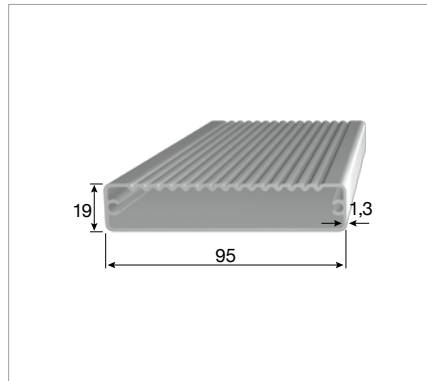
Profil za ladijski pod na terasah P9519
