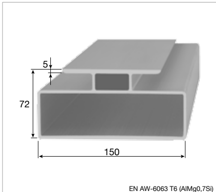
Podlahový profil P15072
