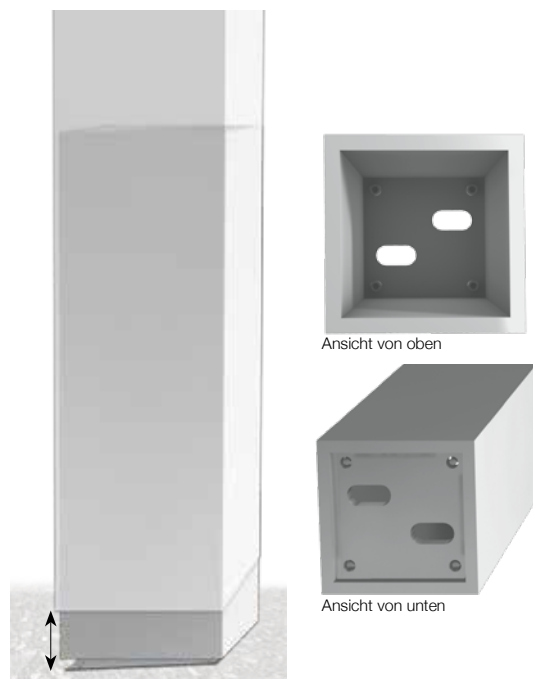
Montagebeispiel mit Zaunsteher scharfkantig
